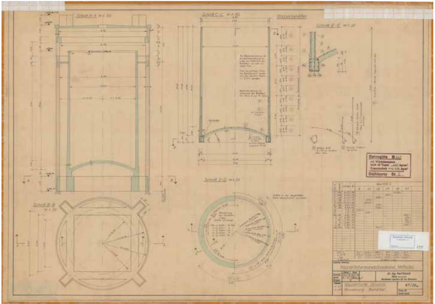
Konstruktionszeichnung Wasserturm Ginnick, März 1953
