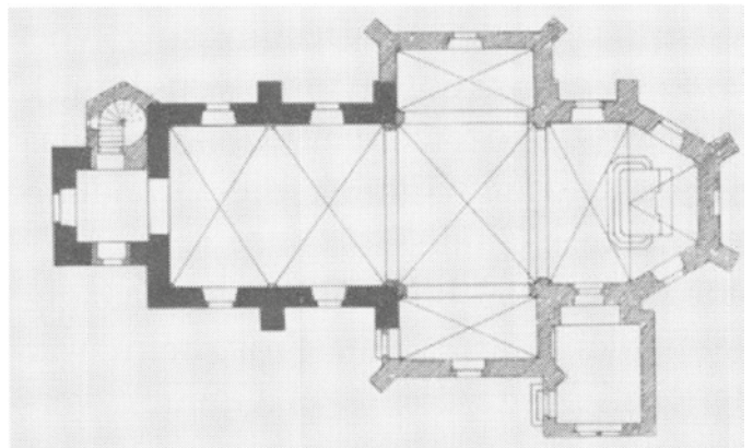
Grundriss der Kirche mit altem Bestand um 1660 und 1720 (dunkle Umrahmung) und der Erweiterung 1897
